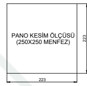
PANO KESİM ÖLÇÜSÜ (250X250 MENFEZ)
